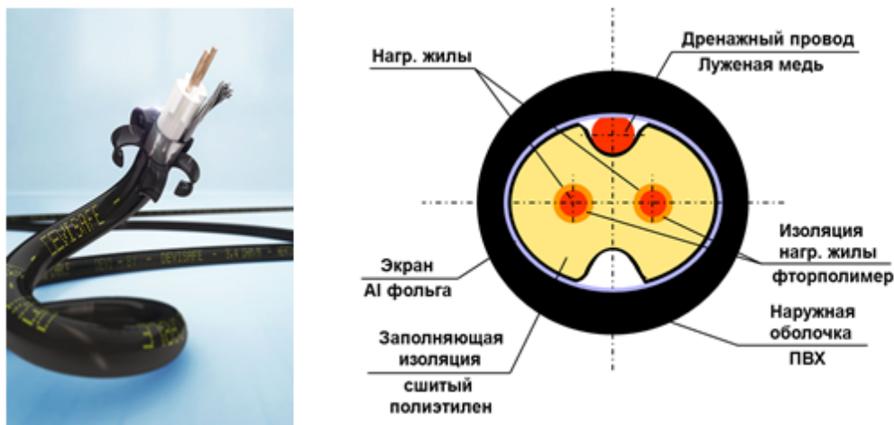
Рис. 2. Устройство нагревательного кабеля ДЕВИ Snow-30Т
